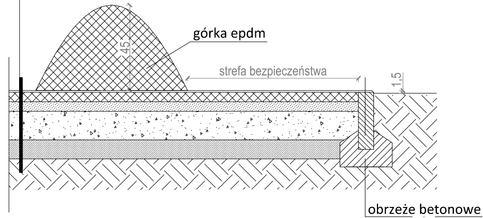
PRZEKRÓJ D-D
