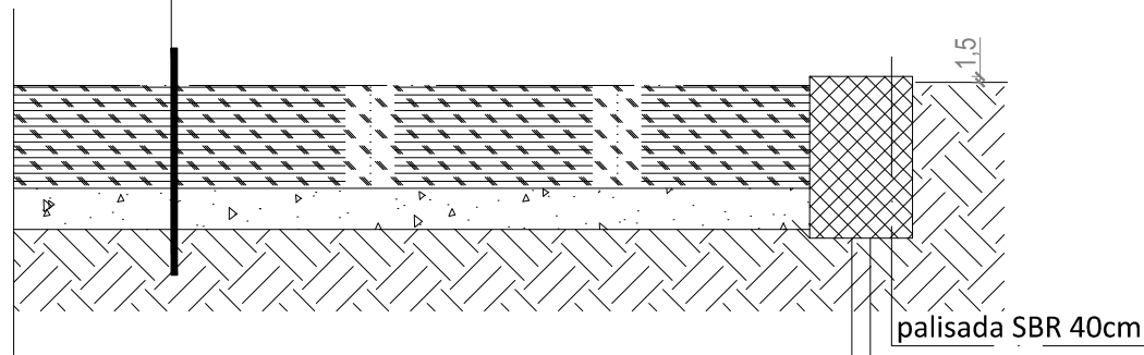
PRZEKRÓJ B-B
