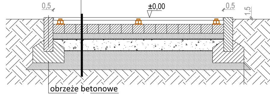
PRZEKRÓJ A-A
