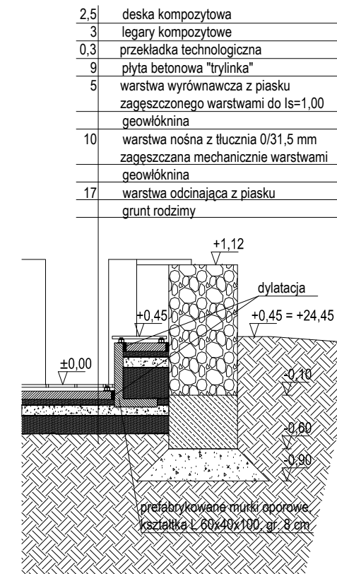
PRZEKRÓJ C-C
