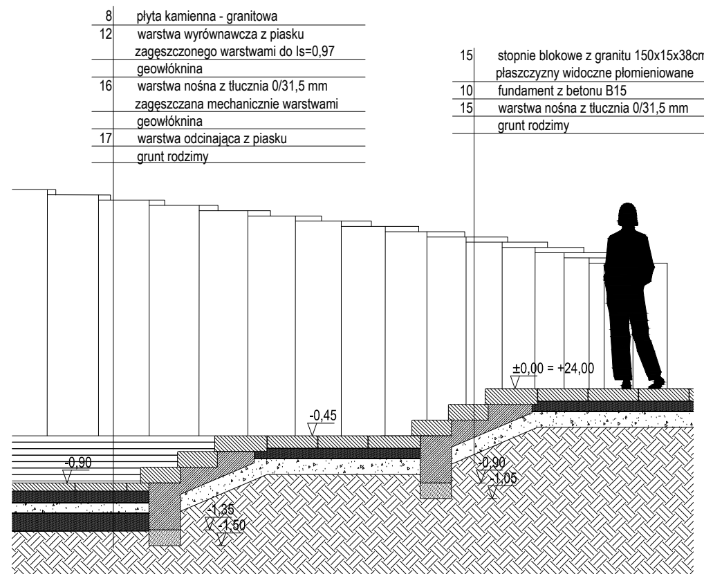
PRZEKRÓJ B-B
